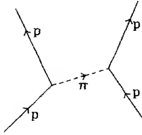
شكل ٩-١٤: بروتونان يتنافران بعضهما من بعض بتبادل بيون.
